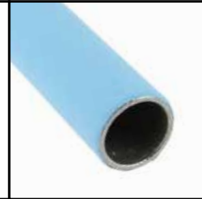
T2-400 KOLOR RURKA STALOWA W KOLORZE (grubość ścianki 1,5 mm, średnica 28,6 mm, długość 4000 mm)
